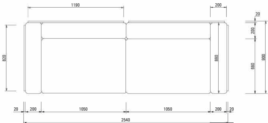
PŮDORYS
