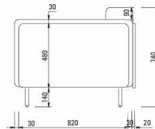
BOČNÍ POHLED
