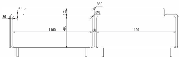
ZADNÍ POHLED
